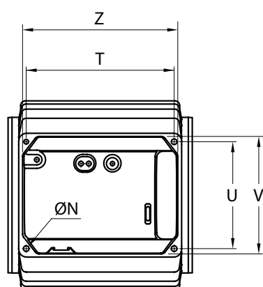
Header MEC 63 B5
