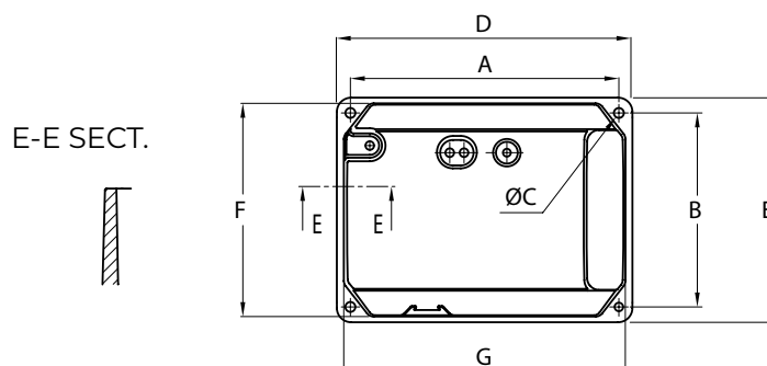
Long header MEC 63 B3-B5
