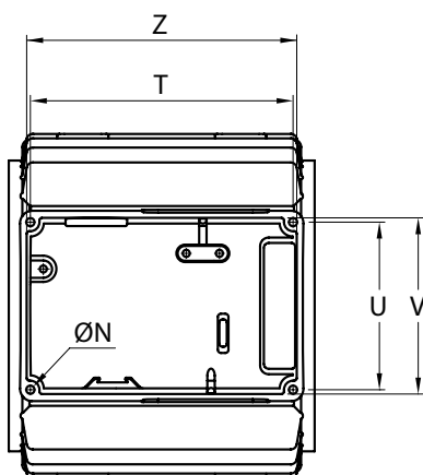
Header MEC 71 B5
