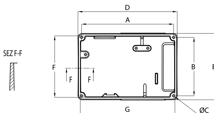
Basetta lunga MEC 71 B3-B5
