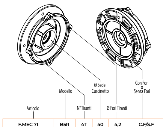
FLANGIA B5 RIDOTTA
